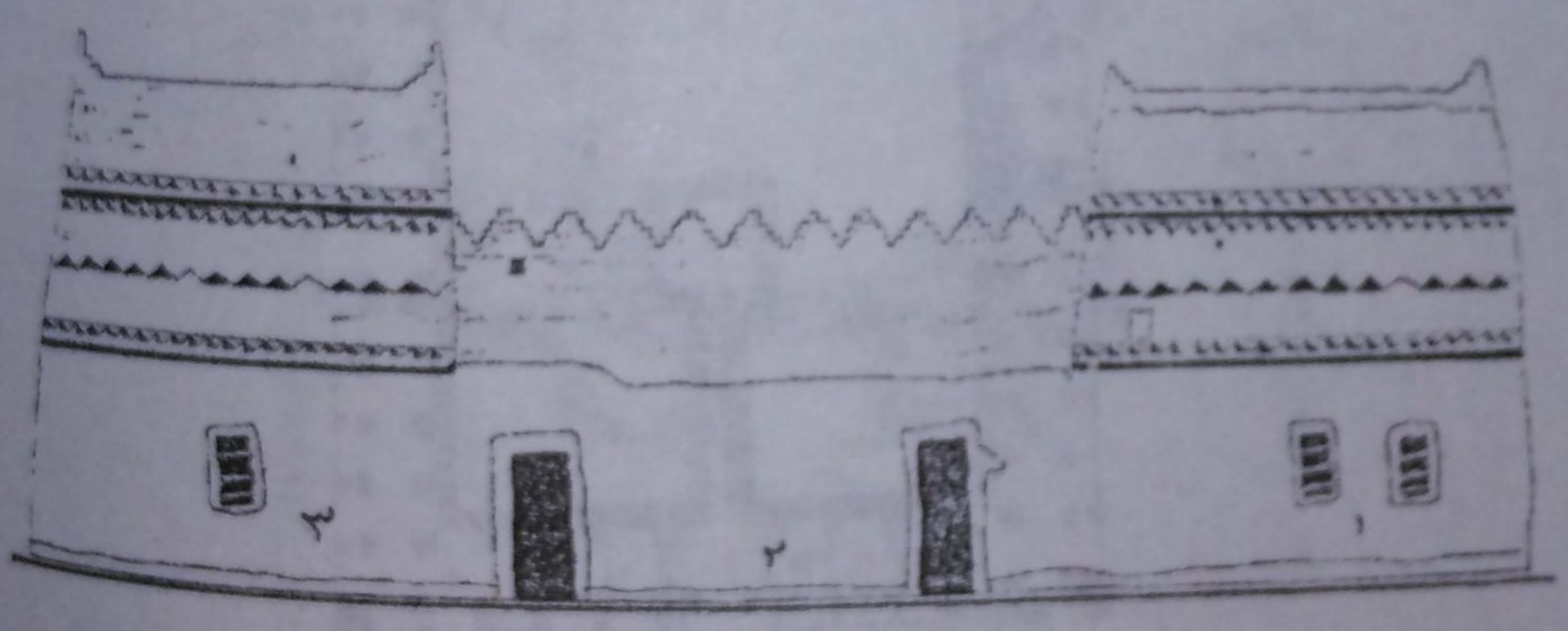
شكل رقم (٥٤) نموذج لمنزل من دور نجد تتضح فيه الثنائية في الواجهات عن الحواس
