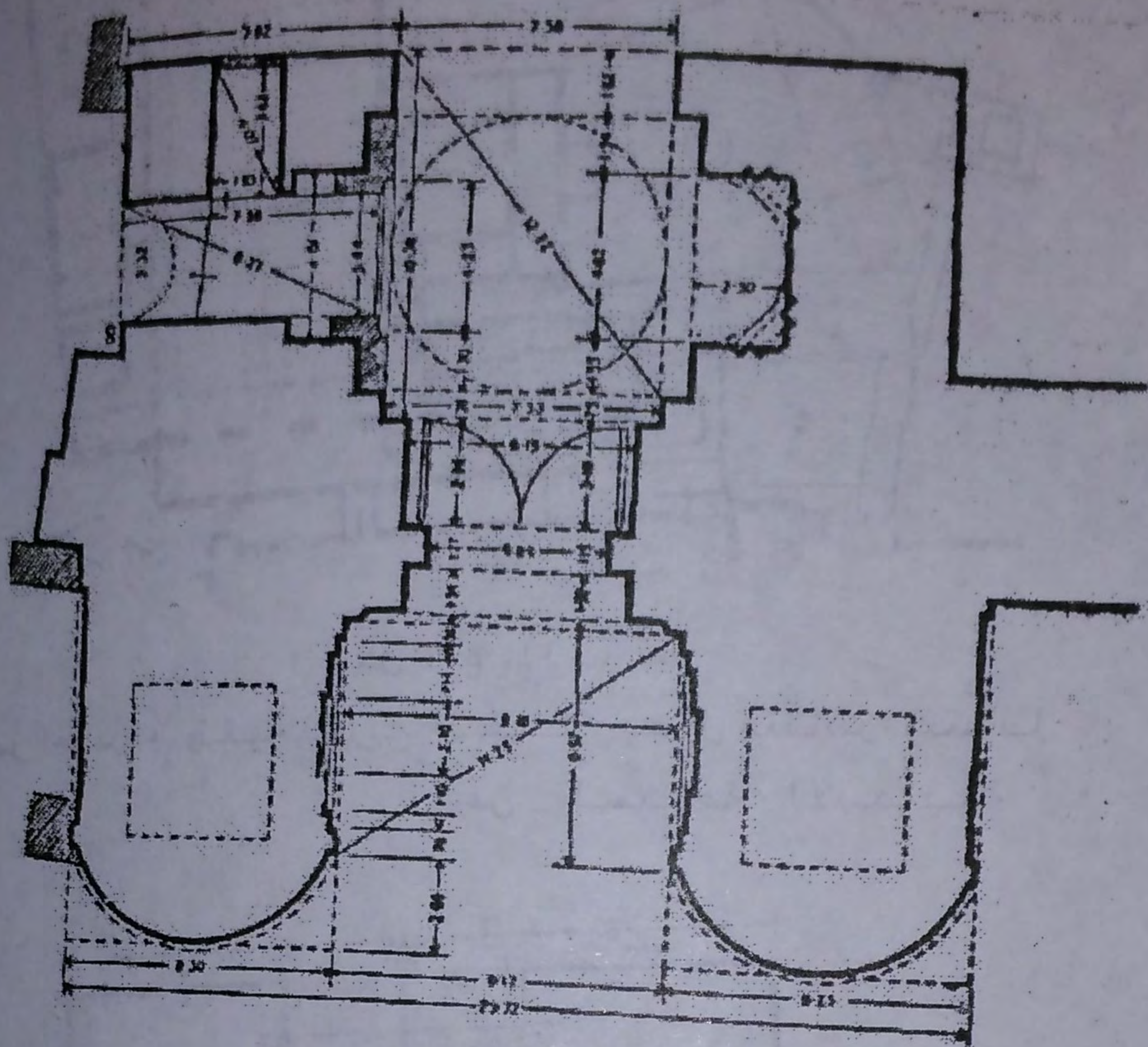
شكل رقم (٨٢) باب زويلة بالسور الجنوبي الفاطمي عن كريزول
