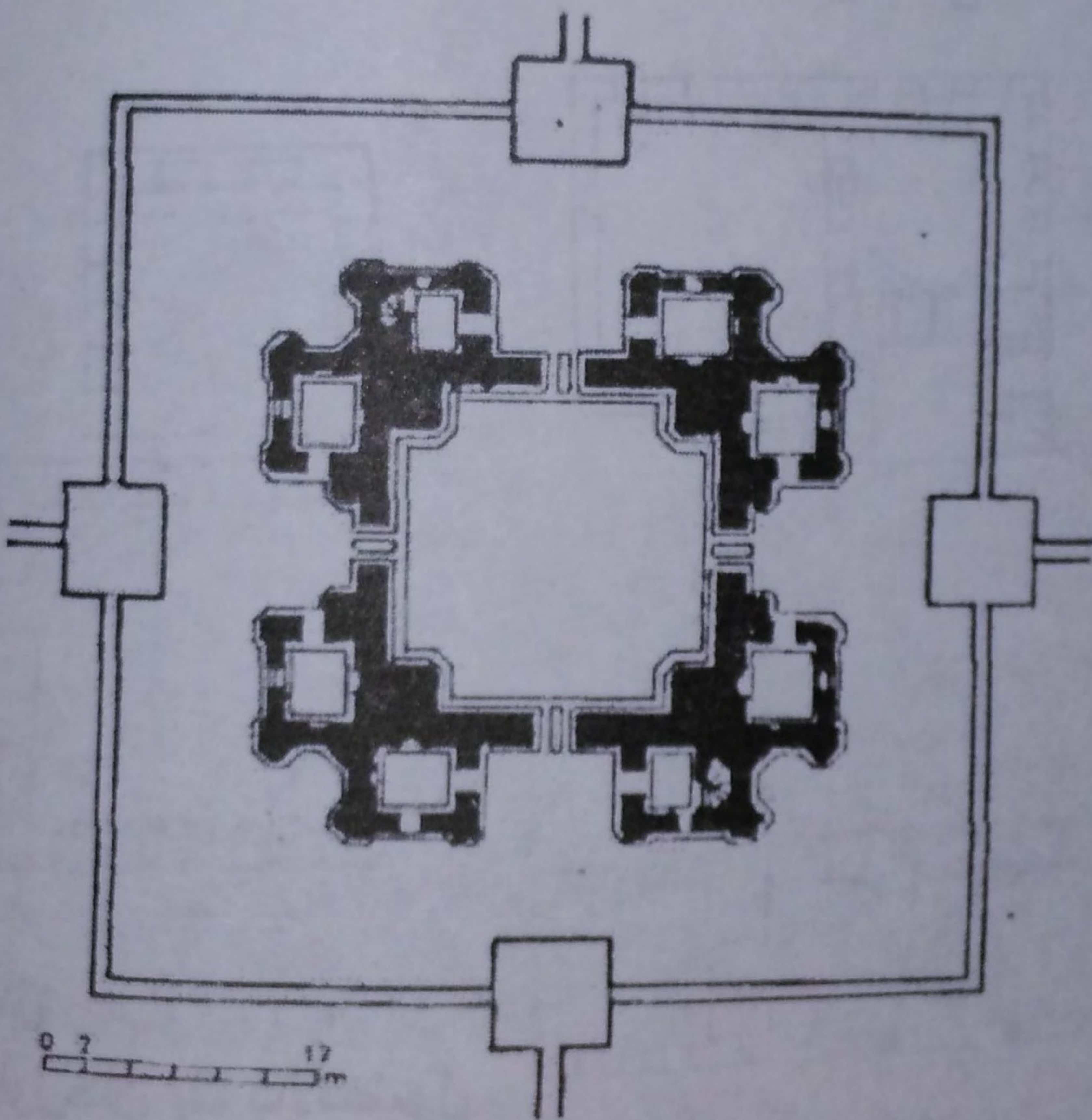
شكل رقم (٥٠) مسقط أفقى لضريح الخواجة رابى فى الهند يتضح فيه ثنائية التخطيط
